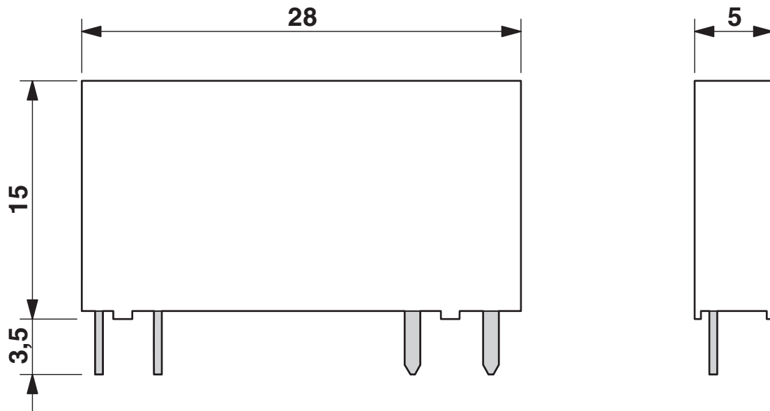
尺寸圖
