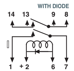
DPST - NO
