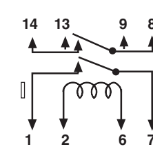
DPST - NO
