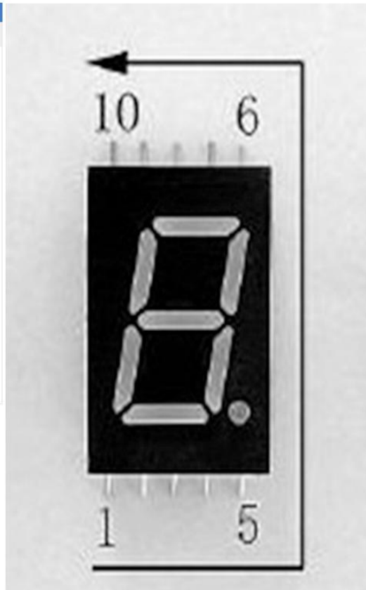
引脚顺序图
