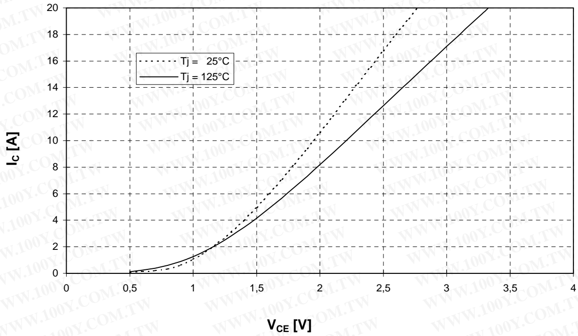
Ausgangskennlinienfeld Brems-Chopper-IGBT (typisch) d = f(V_{CE}) Output characteristic brake-chopper-IGBT (typical) V_{GE} = 15\text{ V}
