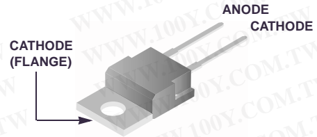
JEDEC TO-220AC
