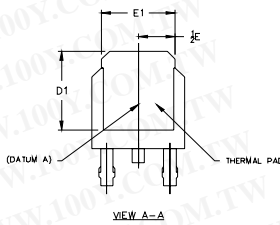
VIEW A-A
