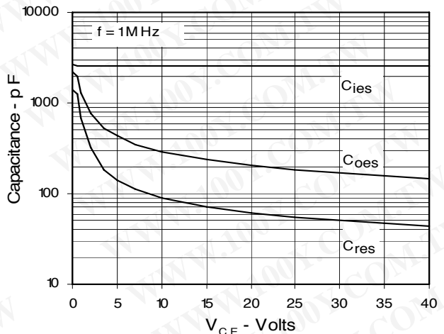
Fig. 12. Capacitance
