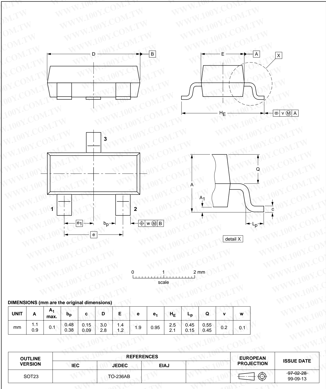
Fig 14. SOT23.
