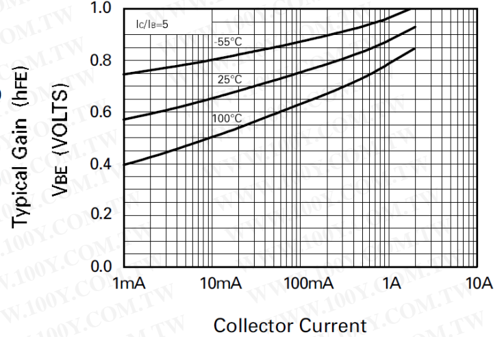
V BE(SAT) vs I C
