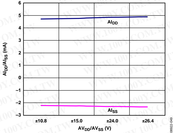
Figure 47. I_{DD}/I_{SS} vs. V_{DD}/V_{SS} , V_{OUT} = 0\text{ V}
