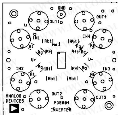
INVERTER SOIC
