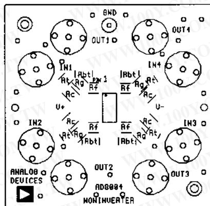
NONINVERTER SOIC
