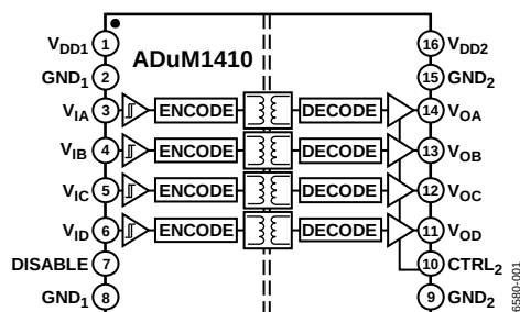
图1. ADuM1410
