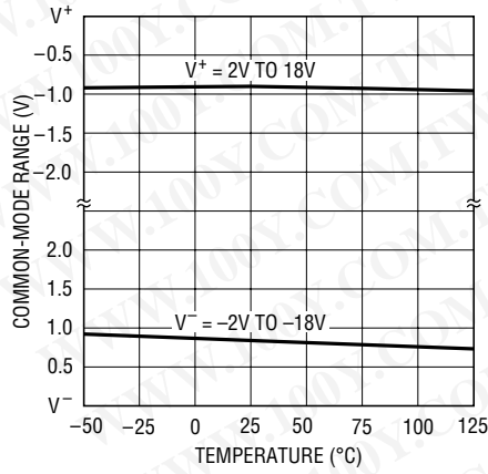
LT1259/60 • TPC16
