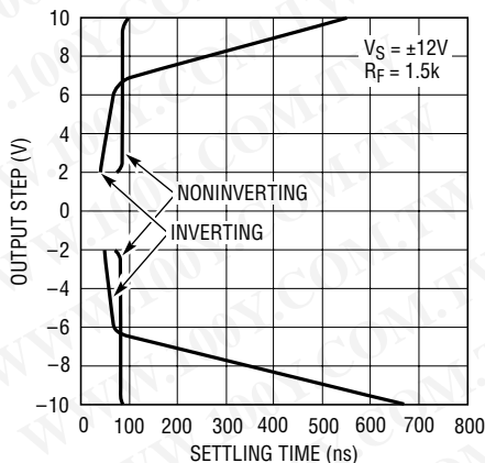
LT1259/60 • TPC17
