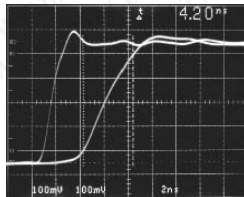
VS = ±15V RF = RG = 1.6k AV = 2 RL = 150Ω
