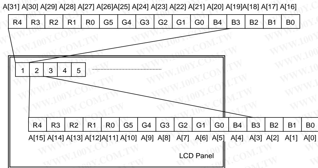
16BPP 5:6:5 Format(Non-Palette)
