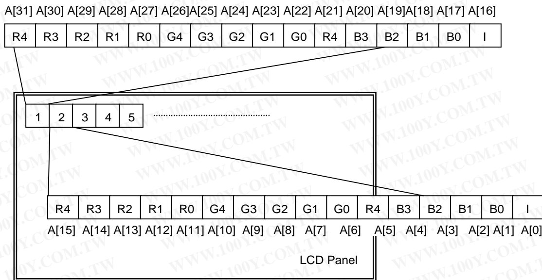
16BPP 5:5:5+1 Format(Non-Palette)
