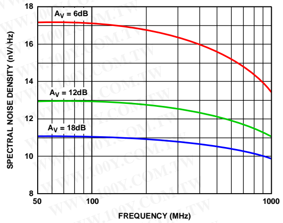
Figure 8. RTO Noise Spectral Density vs. Frequency at AV = 6 dB, AV = 12 dB, and AV = 18 dB
