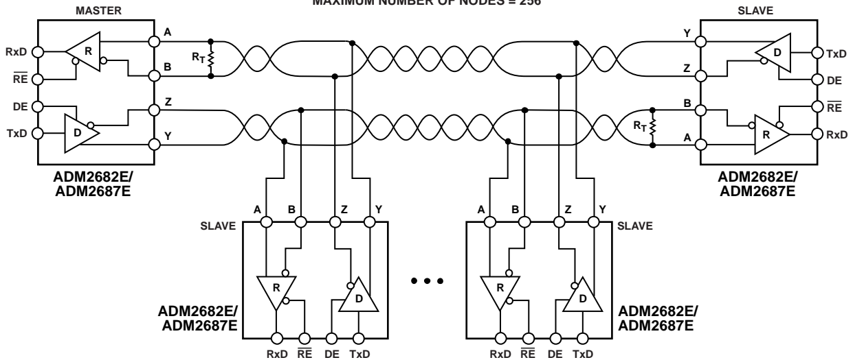
图47. ADM2682E/ADM2687E典型全双工RS-485网络
