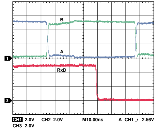
图19. ADM2682E接收器传播延迟
