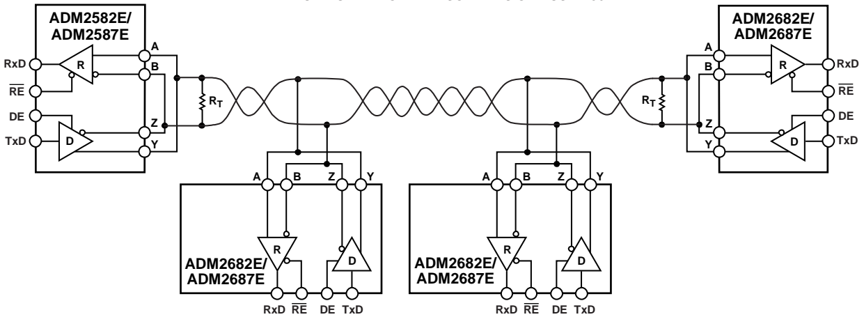
图46. ADM2682E/ADM2687E典型半双工RS-485网络
