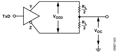
图29. 驱动器电压测量
