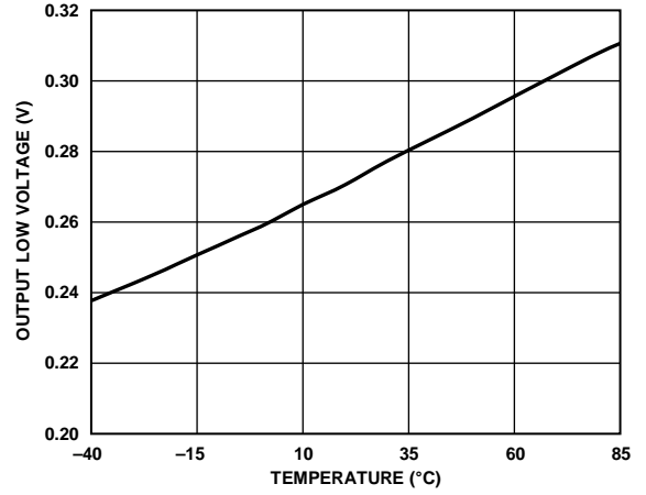
图18. 接收器输出低电压与温度的关系
