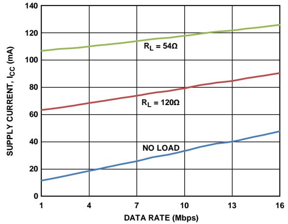
图6. ADM2682E电源电流(I CC )与数据速率的关系 (T A = 25°C, DE = 5 V, V CC = 5 V)
