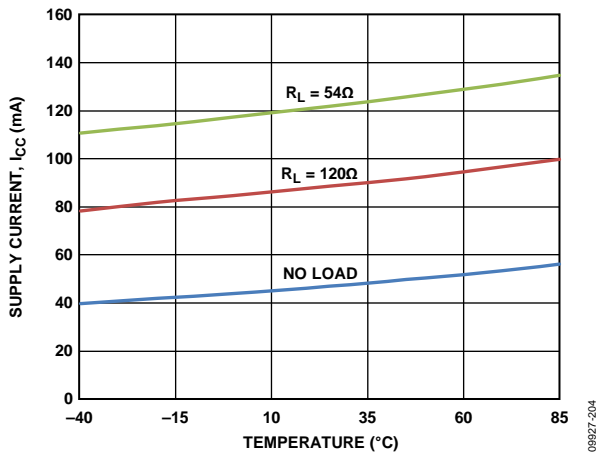
图4. ADM2682E电源电流(I CC )与温度的关系 (数据速率=16 Mbps, DE = 5 V, V CC = 5 V)
