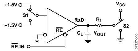
图34. 接收器使能/禁用
