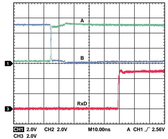
图20. ADM2687E接收器传播延迟
