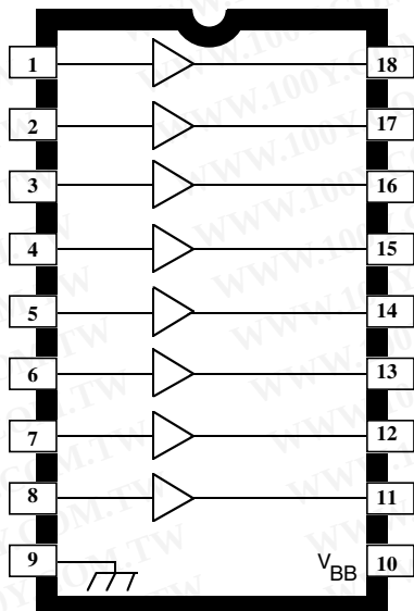
UDN6118A
