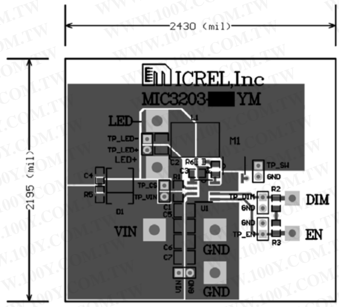
Top Layer
