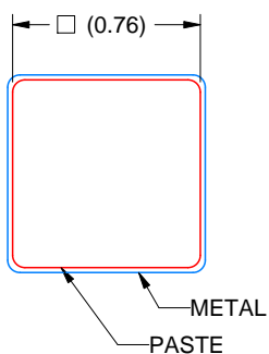
DETAIL A 4X, SCALE: 30X
