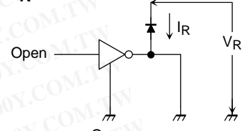
6. I_R
