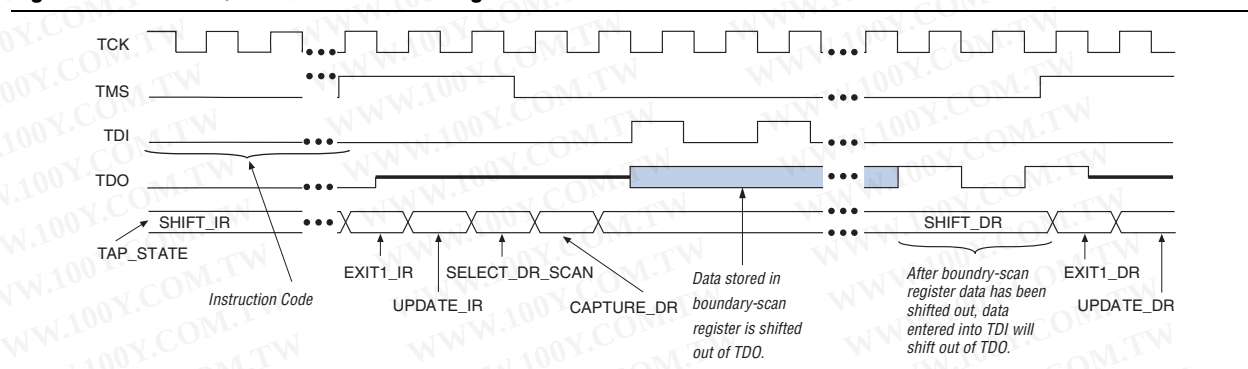
Figure 8-9. SAMPLE/PRELOAD Shift Data Register Waveforms
