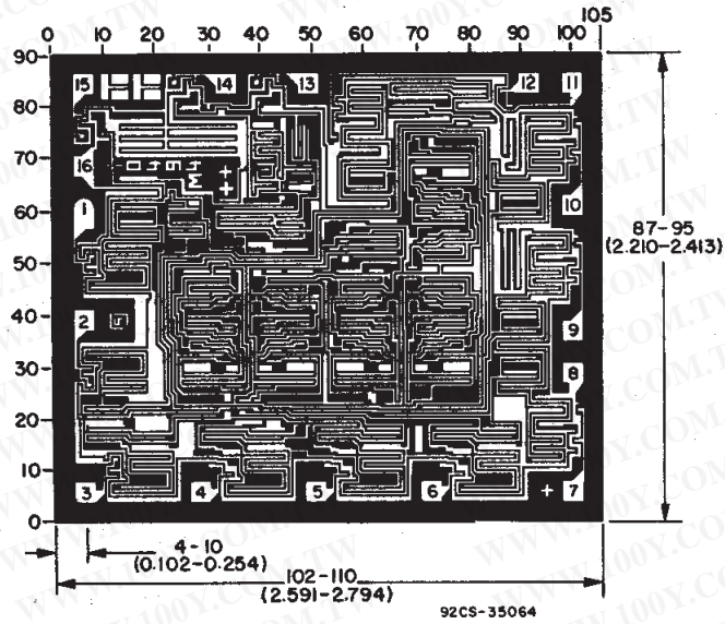
CD4017BH
