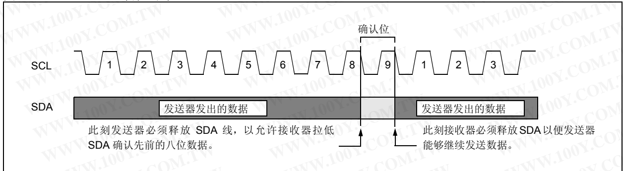
图 5-2: 确认时序
