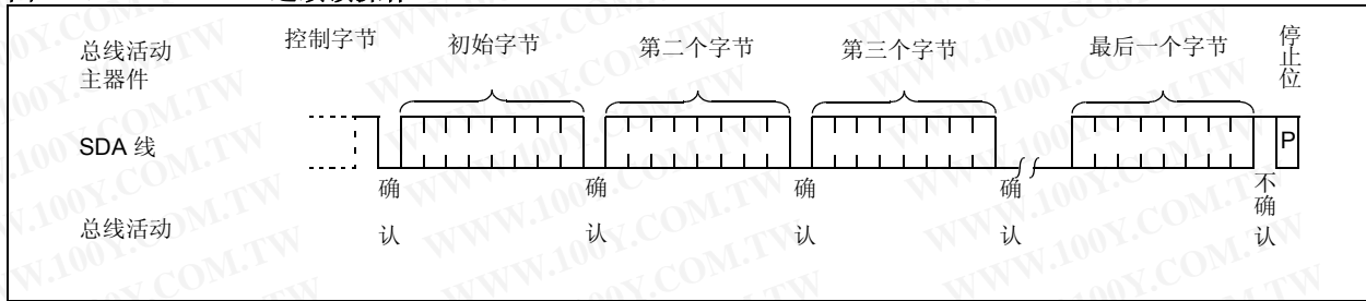
图 8-4: 连续读操作
