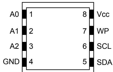
8-pad UDFN
