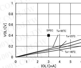
Fig.5 L output voltage VOL,1-IOL1 (VCC=2.5V)
