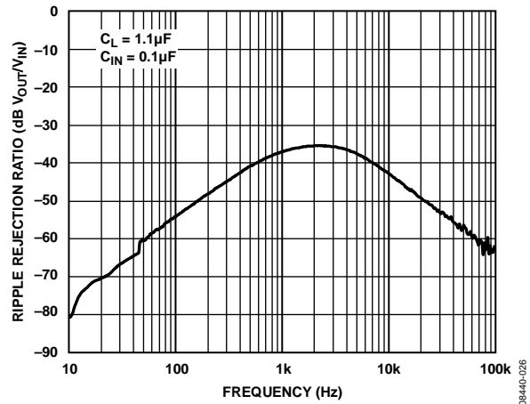
图24. ADR3450纹波抑制比与频率的关系
