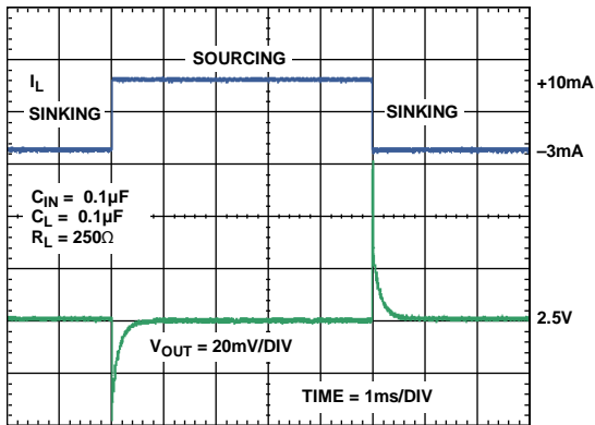
图29. ADR3425负载瞬态响应
