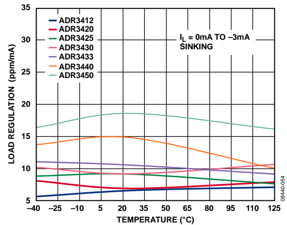
图8. 负载调整率与温度的关系(吸电流)
