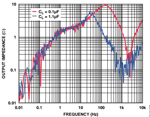
图35. ADR3450输出阻抗与频率的关系
