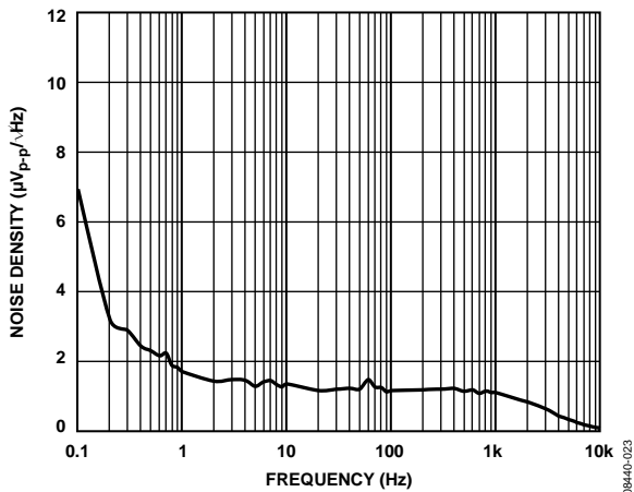
图17. ADR3425输出噪声频谱密度
