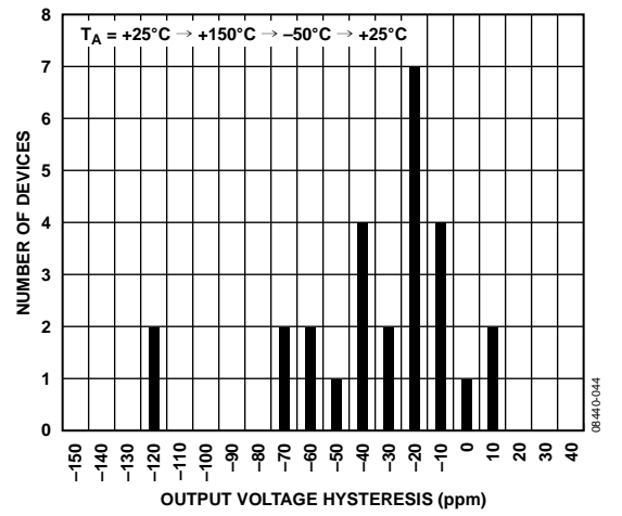
图37. ADR3450热致输出电压迟滞分布图
