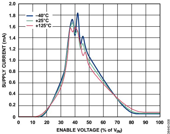
图34. 电源电流与ENABLE引脚电压的关系
