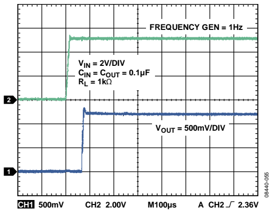
图11. ADR3412启动(开启建立)时间
