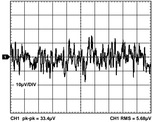
图21. ADR3450输出电压噪声(0.1 Hz至10 Hz)
