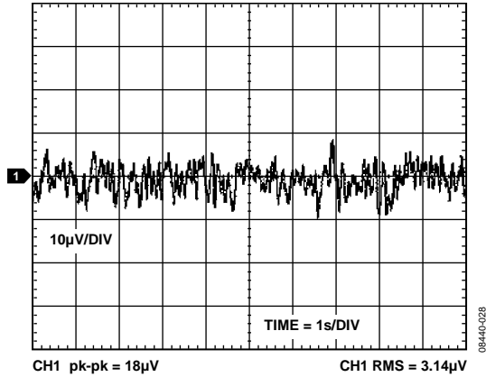
图15. ADR3425输出电压噪声(0.1 Hz至10 Hz)
