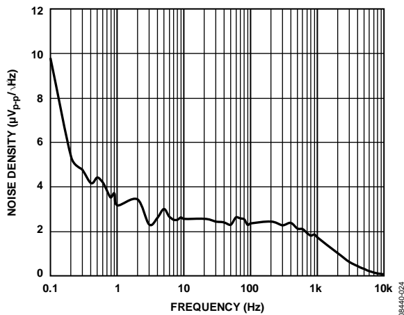
图23. ADR3450输出噪声频谱密度
