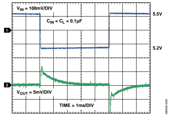
图31. ADR3450线路瞬态响应
