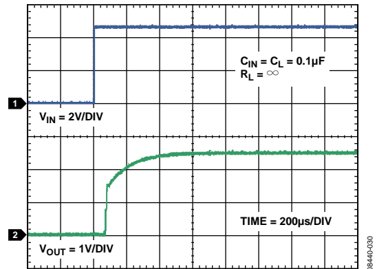
图19. ADR3425启动响应
