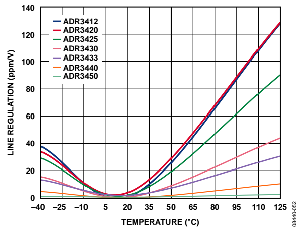
图14. 电压调整率与温度的关系
