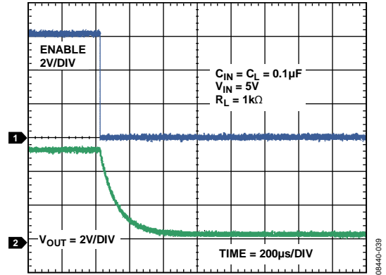
图30. ADR3450关断响应
