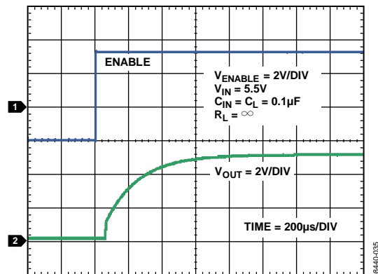
图26. ADR3450从关断状态重启的响应性能
