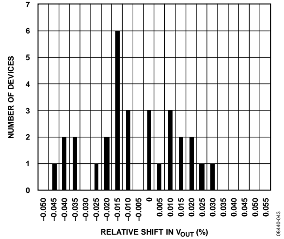
图36. 回流后的输出电压漂移分布图(SHR漂移)
