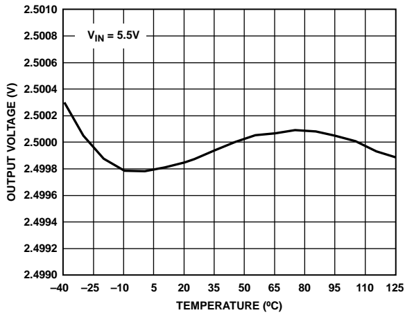
图3. ADR3425输出电压与温度的关系
