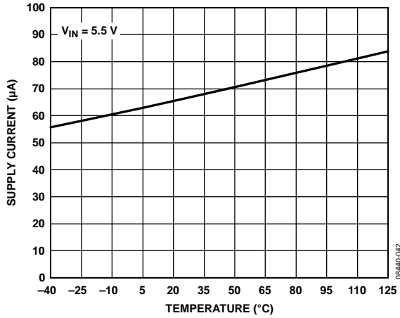
图33. 电源电流与温度的关系
