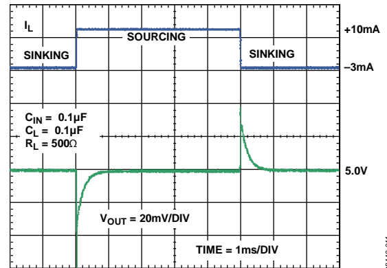
图32. ADR3450负载瞬态响应
