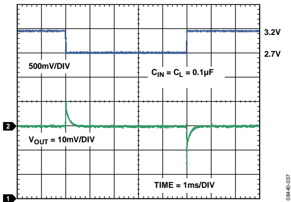
图28. ADR3425线路瞬态响应
