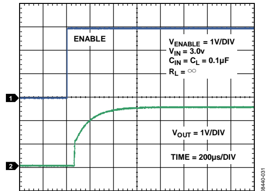
图20. ADR3425从关断状态重启的响应性能
