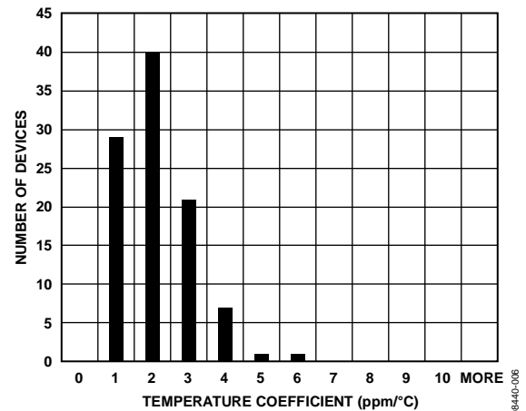
图7. ADR3450温度系数分布图
