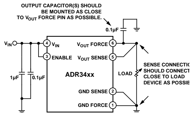
图41. 开尔文连接应用示例
