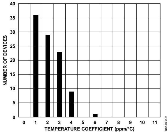
图4. ADR3425温度系数分布图
