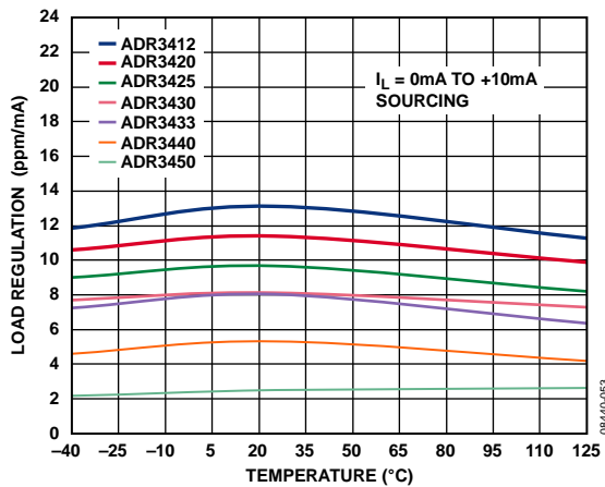
图5. 负载调整率与温度的关系(源电流)
