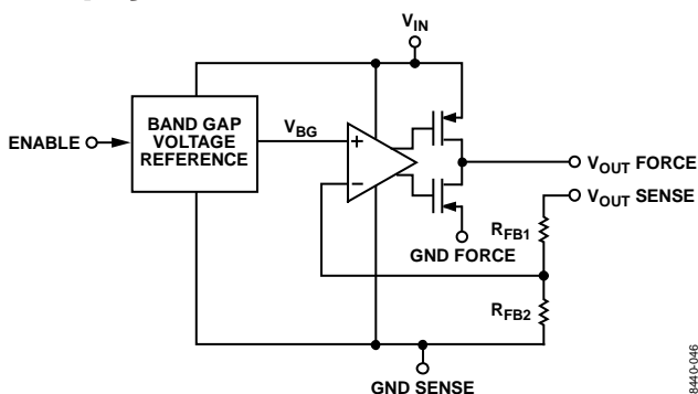
图39. 功能框图
