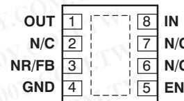
DRB PACKAGE 3mmx 3mm SON (TOP VIEW)
