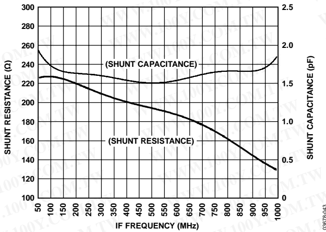
Figure 43. Input Impedance of Mixer Input vs. F_{IF} , V_{GIN} = 0.7 V , V_{POS} = 5 V
