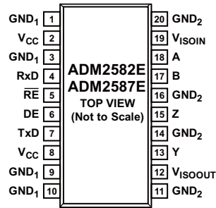
图2. 引脚配置
