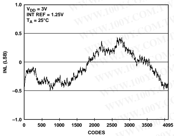
Figure 20. INL AD5628-1
