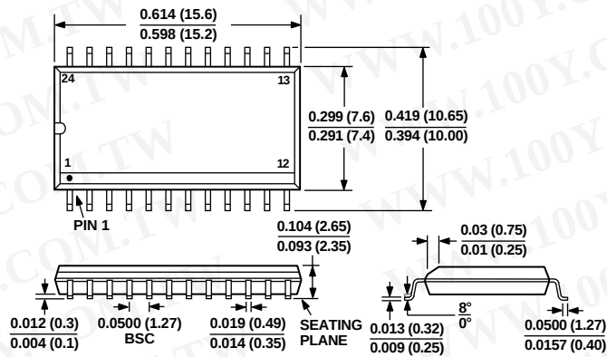
SOIC (R-24)
