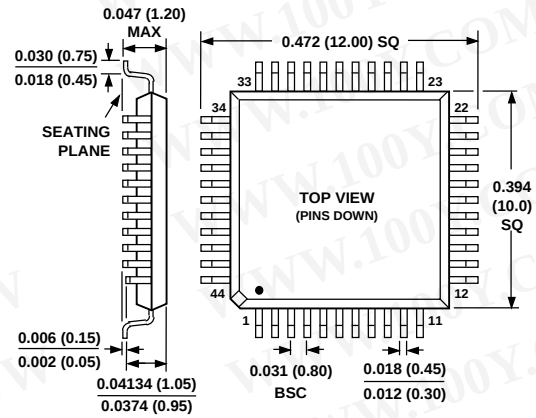
TQFP (SU-44)
