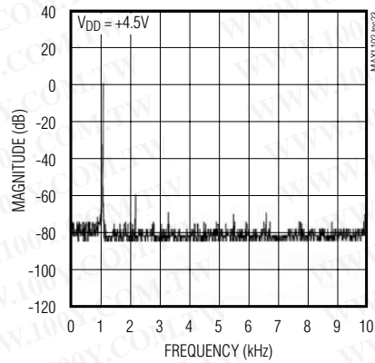
DAC FFT
