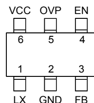
SOT-23-6
