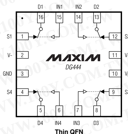
Thin QFN
