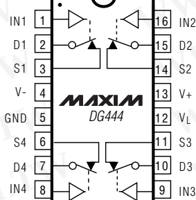
DIP/SO
