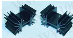
Part No. 1756 Product No. AK-122-25mm+Pin 說明 散熱片 黑色 長度 25mm Size: 42W*25H*50Dmm
