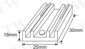
Part No. 16966 Product No. AK-146-30mm+Pin 說明 散熱片 白色 Size 30*25*18mm
