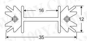
Part No. 5990 Product No. AK-132-24mm+Pin 說明 散熱片 銀色 長度 24mm Part No. 53986 Product No. AK-132-25mm+Pin 說明 散熱片 黑色 長度 25mm
