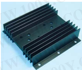
Part No. 1747 Product No. AK-109-100mm 說明 散熱片 黑色 長度 100mm Part No. 1748 Product No. AK-109-200mm 說明 散熱片 黑色 長度 200mm
