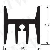
Part No. 16964 Product No. AK-147-25mm 說明 散熱片 白色 Size 25*14.5*17mm
