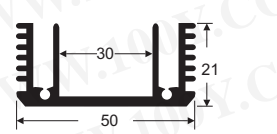
Part No. 5991 Product No. AK-141-50mm 說明 散熱片 黑色 長度 50mm
