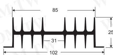
Part No. 29436 Product No. AK-106-100mm 說明 散熱片 鋁本色 長度 100mm
