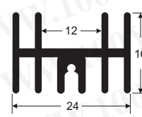
Part No. 5991 Product No. AK-141-50mm 說明 散熱片 黑色 長度 50mm
