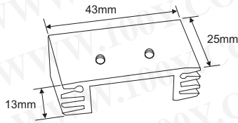
Part No. 8354 Product No. AK-087-25mm 說明 散熱片黑色
