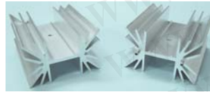
Part No. 30865 Product No. AK-122-50mm+Pin 說明 散熱片 長度 50mm
