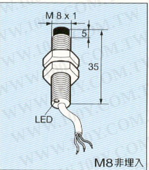
M8非埋入
