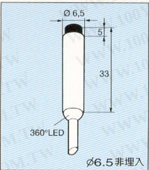
φ6.5非埋入
