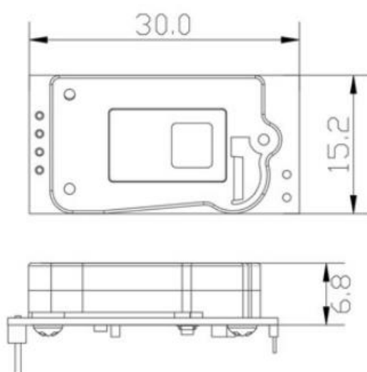
ACD10 传感器结构尺寸图 (单位: mm)
