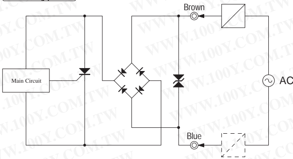
AC type
