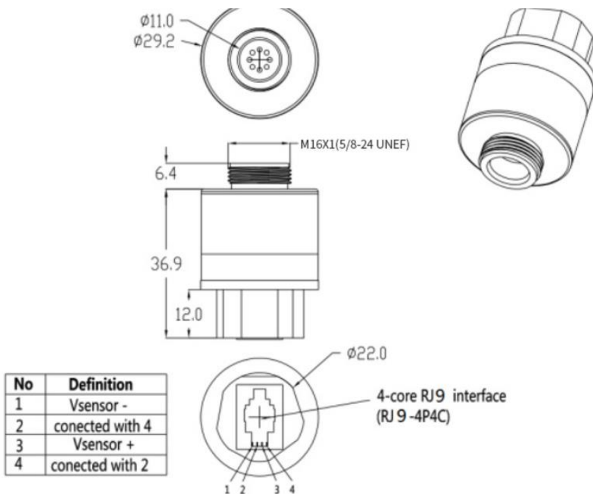
AO-07氧气传感器外形尺寸图
