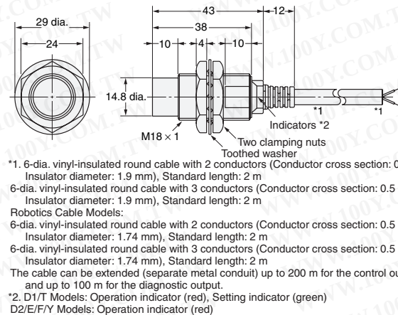
Diagram 15 E2E-X14MD□/E2E-X10ME□/F□ E2E-X10MY□
