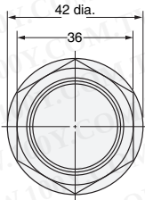
Diagram 36 E2E-X20MD1-M1GJ E2E-X20MD1-M1TGJ
