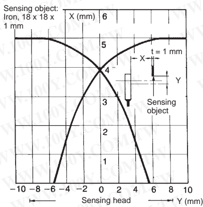
TL-W5
