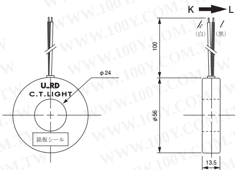
〔外形図〕 CTL-24 シリーズ
