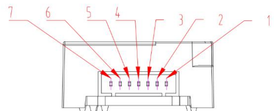
图 4 管脚定义图
