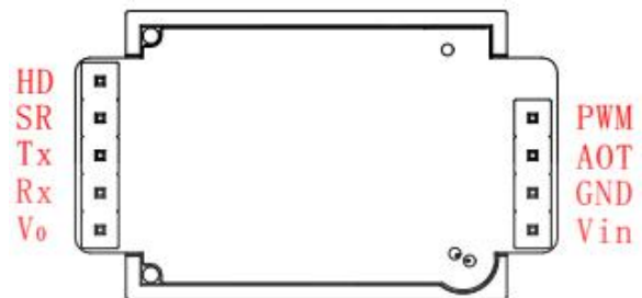
图 3 引脚图
