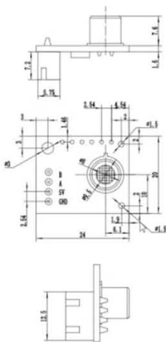
图 1: 模组结构图
