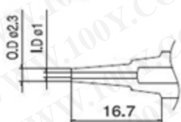
N1-L10 吸咀 1.0mm 長
