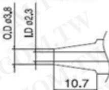
N1-23 吸咀 2.3mm
