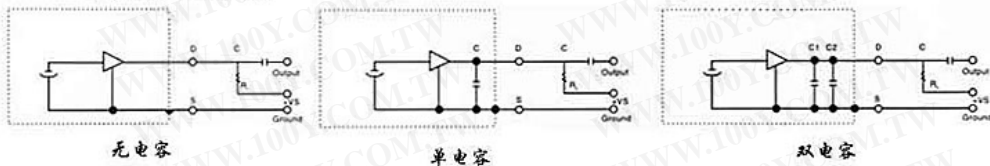
測試電路圖
