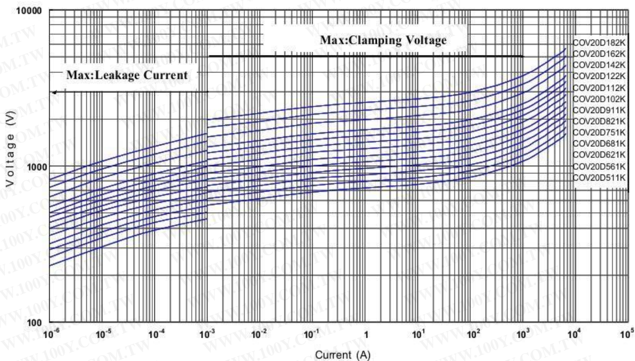
V - I (COV20D511K to COV20D182K)
