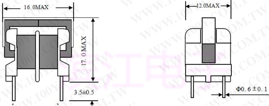
UU9.8立式尺寸图
