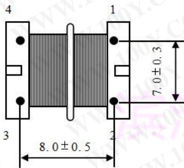
UU9.8立式尺寸图
