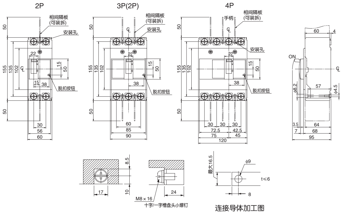
端子部详图
