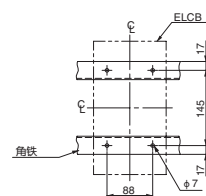
安装开孔尺寸(角铁安装时)
