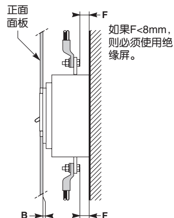
MCCB与正面面板之间的最小距离
