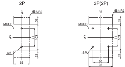
安装开孔尺寸(面板安装时)
