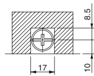
端子部详图
