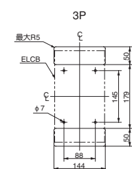
安装开孔尺寸(面板安装时)
