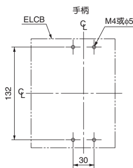
安装开孔尺寸
