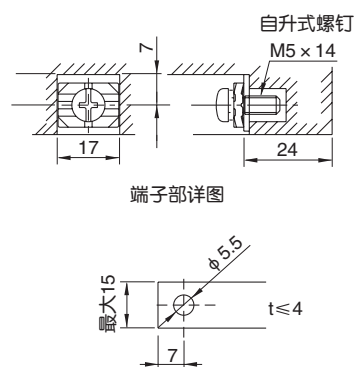
连接导体加工图
