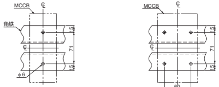
安装开孔尺寸(角铁安装时)
