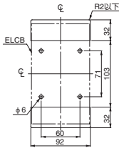
安装开孔尺寸(面板安装时)
