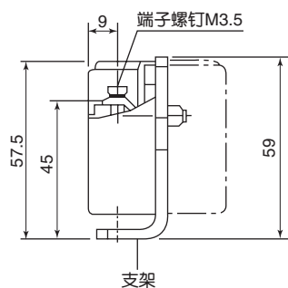
P向视图
