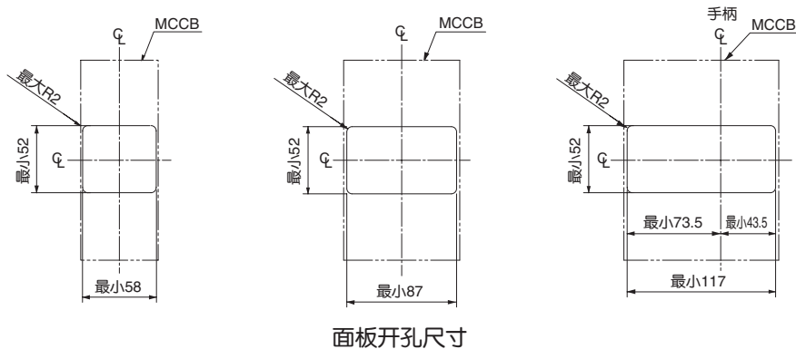
安装开孔尺寸
