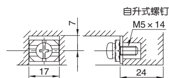
端子部详图
