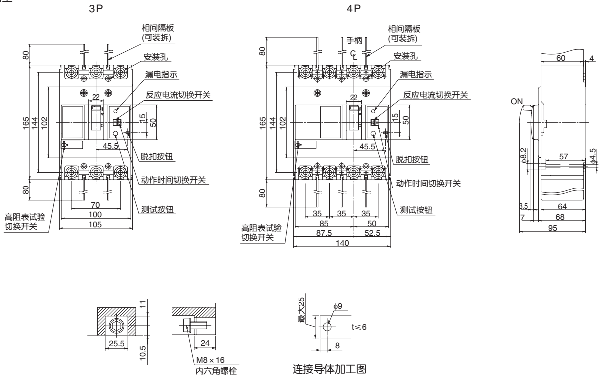
端子部详图
