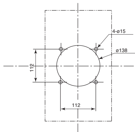
· 面板开孔尺寸图
