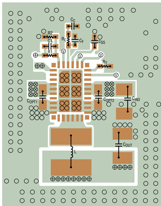
b) LT8646S
