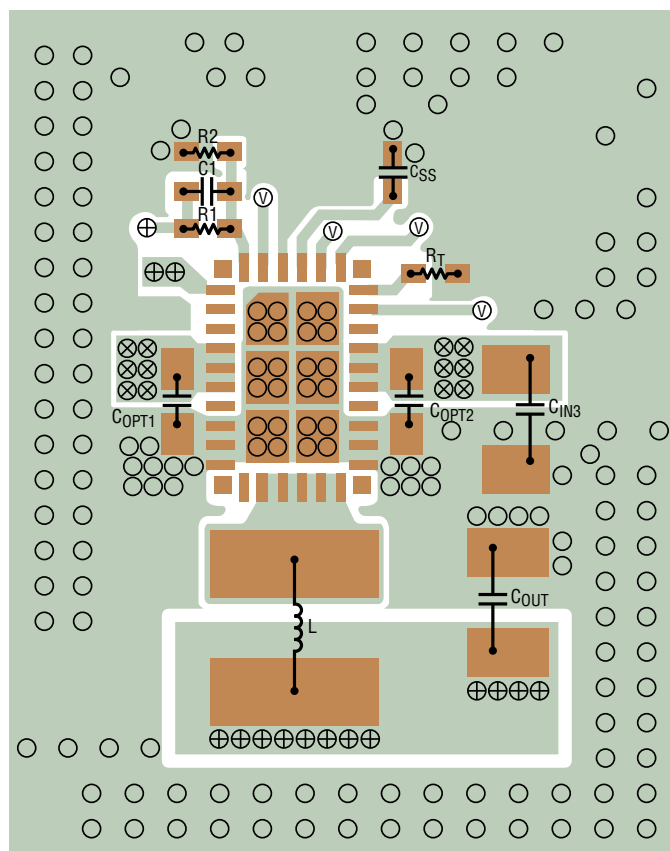
a) LT8645S
